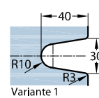
Glasbearbeitung
