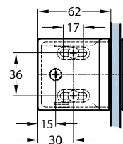
Für 8 mm Glas
